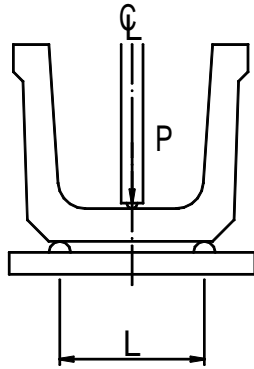
P: 試験荷重 L: 試験用スパン
