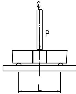
P:試験荷重 L:試験用スパン
