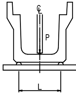
P: 試験荷重 L: 試験用スパン
