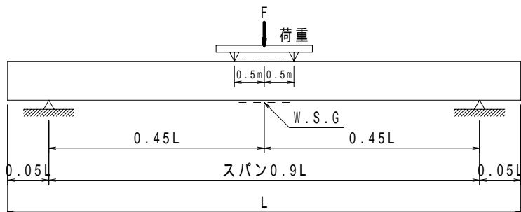
図 1 載荷方法
